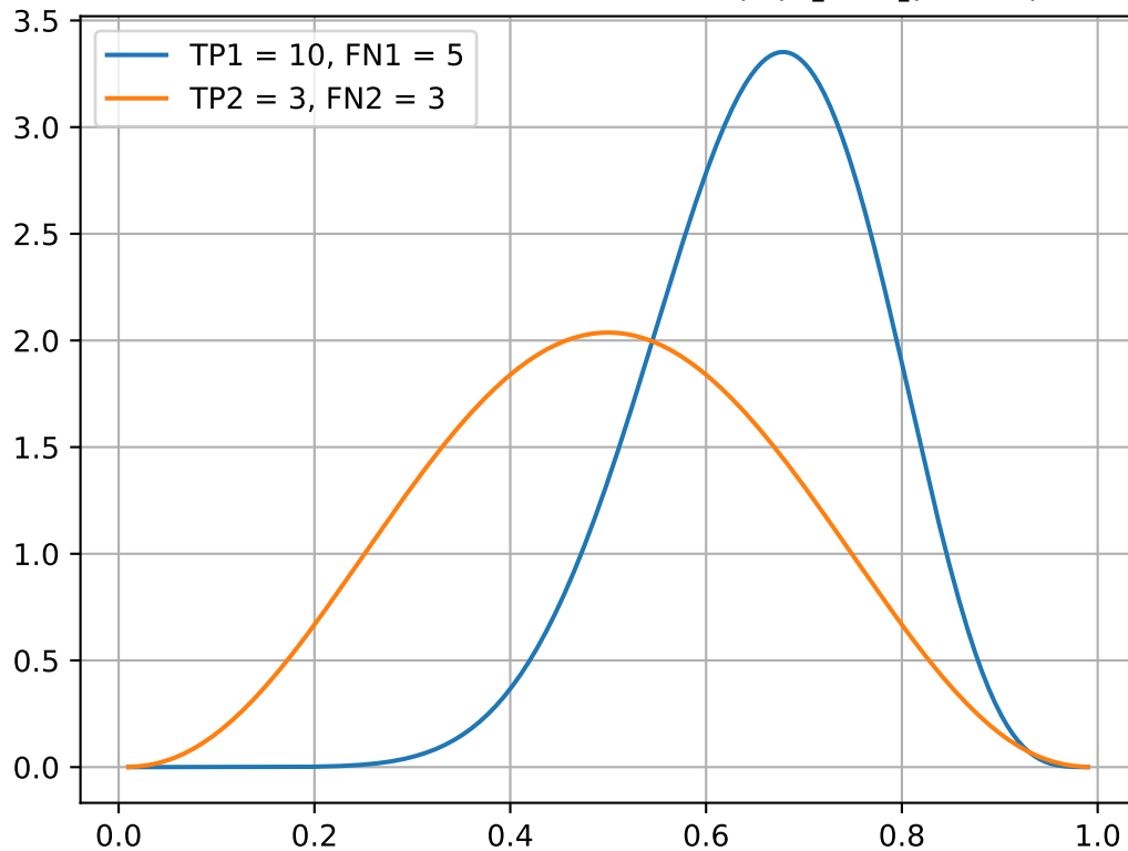
Posterior Recall - Monte Carlo - ( \mathbb{P}(R_2 > R_1) : 24%)
