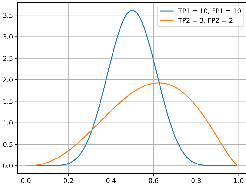
Posterior Precision - Monte Carlo - ( \mathbb{P}(P_2 > P_1) : 66%)
