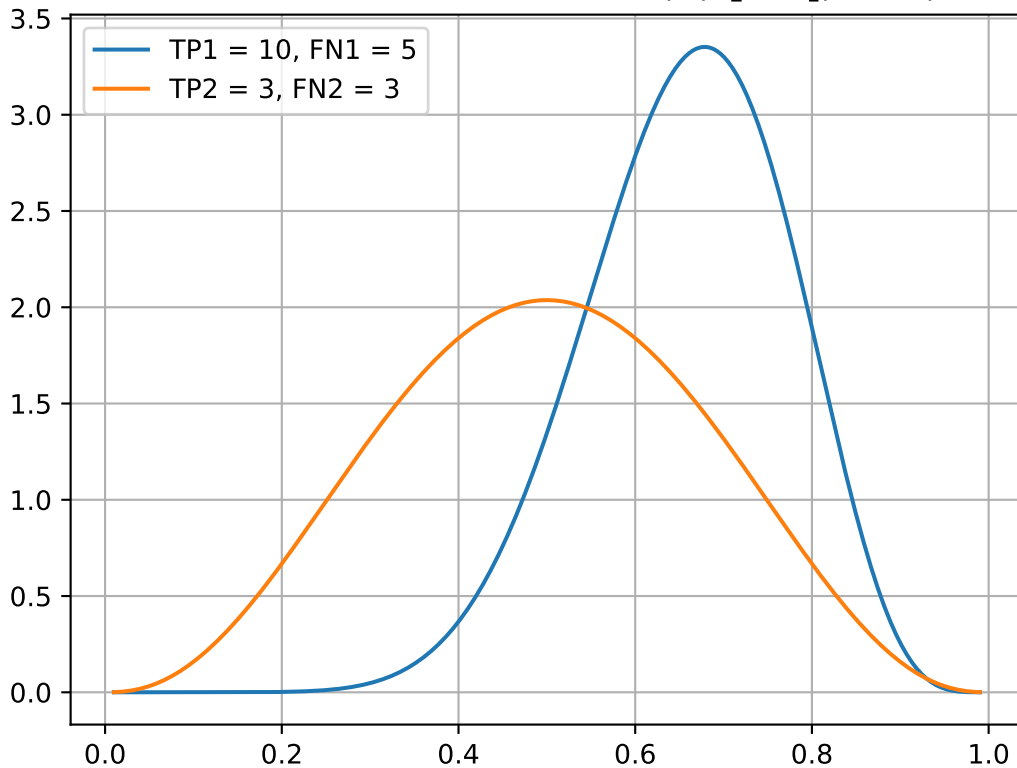
Posterior Recall - Monte Carlo - ( P(R_2 > R_1) : 24%)
